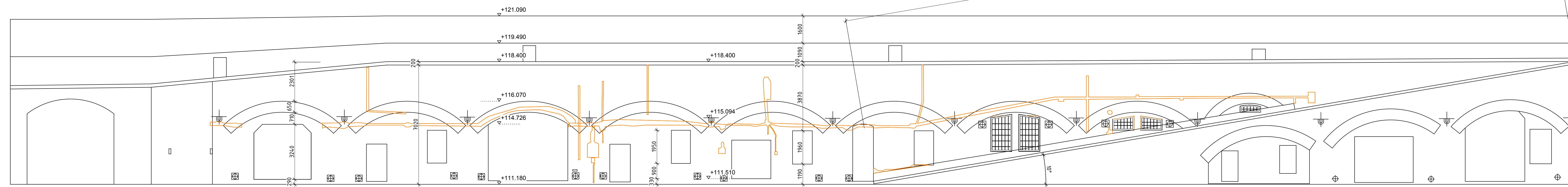
Pohľad - jestvujúci stav
